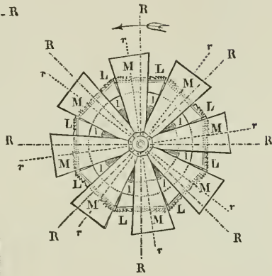
Plan Fig. 40.
