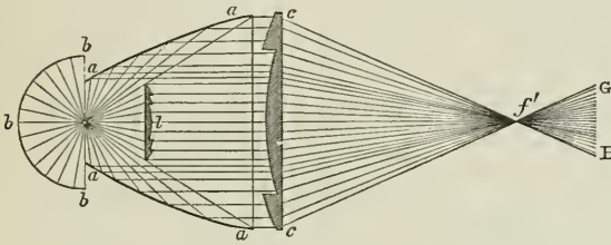
Section Fig. 79.
