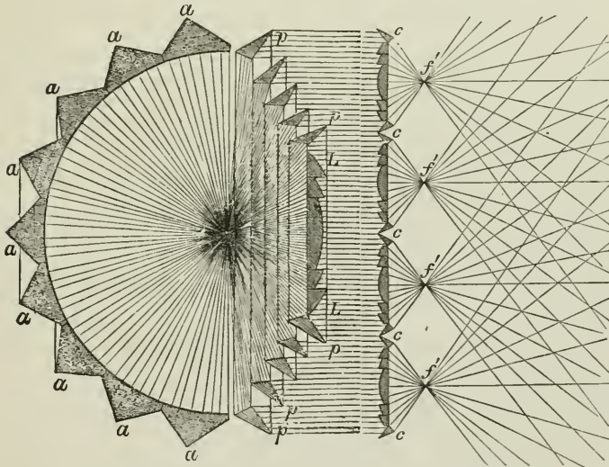
Middle Horizontal Fig. 81.
