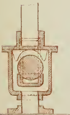
BALL VALVES F. F.
