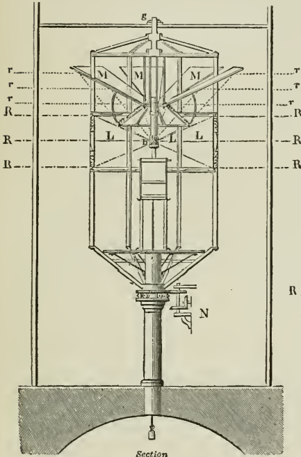
Section Fig. 39.
