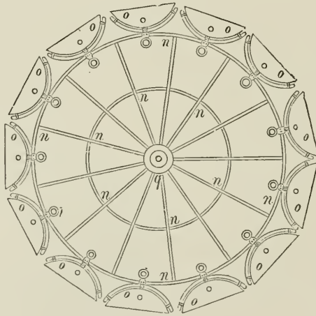
Plan Fig. 22.
